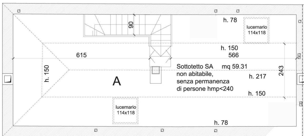
PIANTA PIANO SOTTOTETTO
